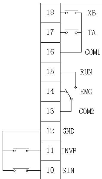
图 6 端子 (10~18)
