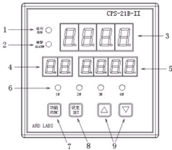
图 3 整机前视图
